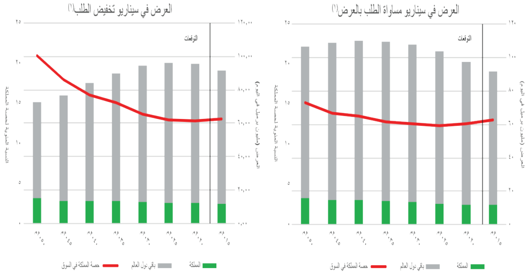
الشكل ٧: العرض الضعفي والمتوقع على المنتجات المكررة حسب المنطقة خلال الفترة من عام ٢٠١٥م إلى عام ٢٠٥٠م
