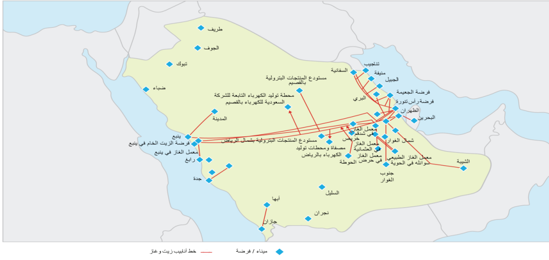
الشكل ١٧: مواقع البنية التحتية لمعالجة النفط الخام للشركة كما في ٣١ ديسمبر ٢٠١٨م
