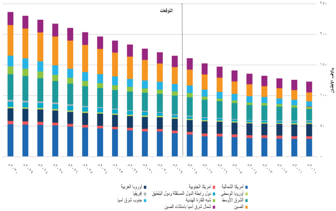
الشكل ١٠: الطلب الفعلي والمتوقع على الإيثيلين عالمياً حسب المنطقة خلال الفترة من عام ٢٠١٠م إلى عام ٢٠٣٠م
